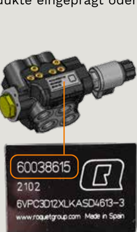
Q-Serie: 3. Steuerkreis-Typenschild
