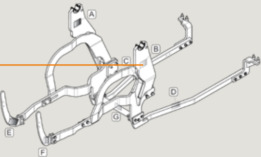
Aufkleber mit Teilenummer auf den Teilen der Anbaukonsole
